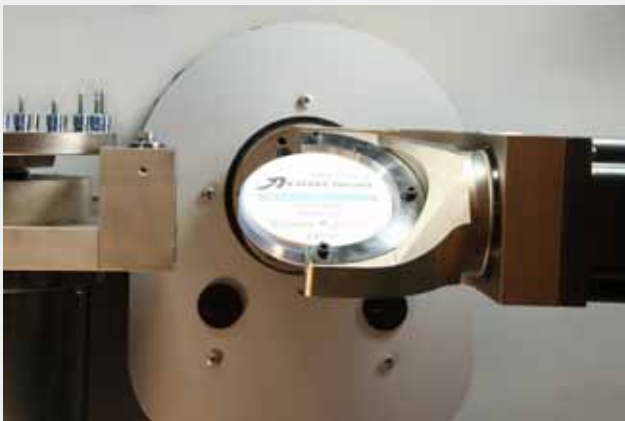
Disco in zirconia posizionato nella pinza a C
