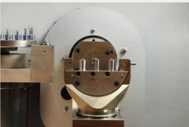
Attrezzatura porta premilled posizionata nella pinza a C
